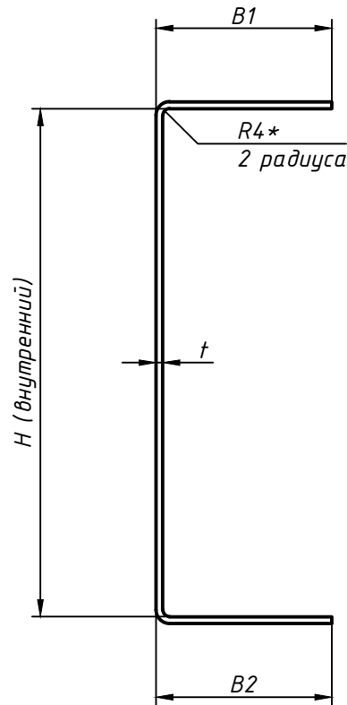
Рисунок А1. - Поперечное сечение профиля ВП U (100-400) xVx t . * - размеры для справок
