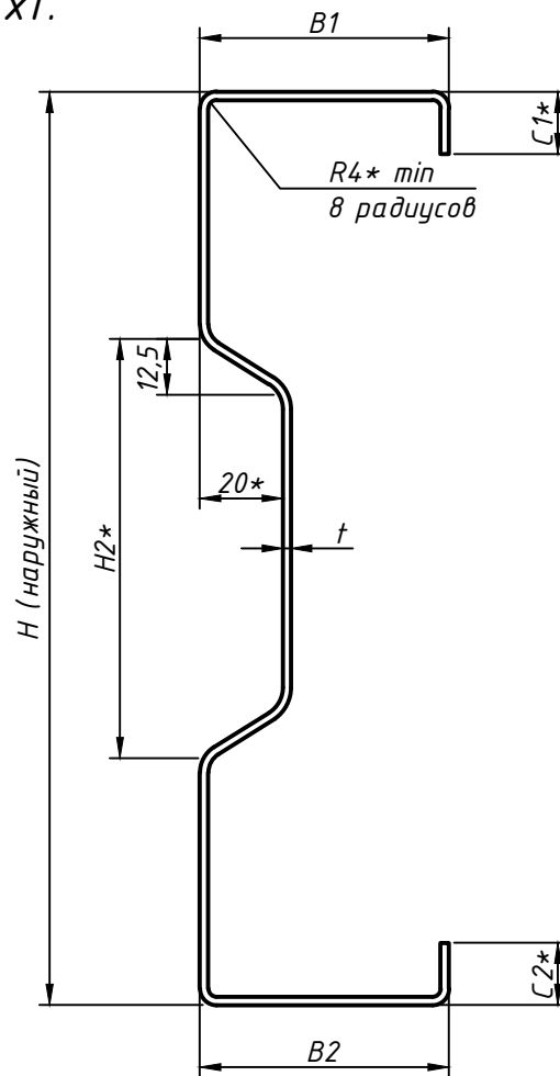
Рисунок А3. - Поперечное сечение профиля ВП \Sigma (200-400) xВxСxt. * - размеры для справок
