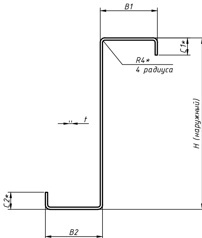
Рисунок А5. - Поперечное сечение профиля ВП Z2 (100-400) хВхСхt. * - размеры для справок
