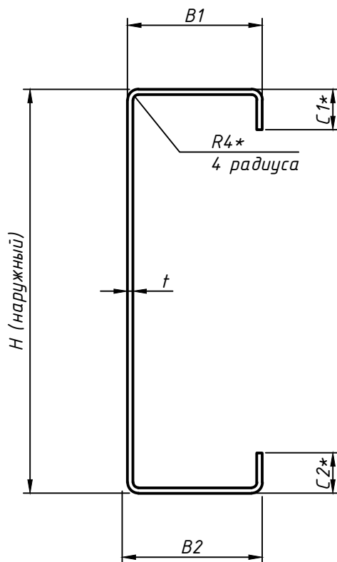
Рисунок А2. - Поперечное сечение профиля ВП С (100-400) хВхСхt. * - размеры для справок
