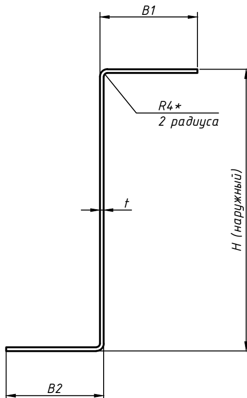
Рисунок А4. - Поперечное сечение профиля ВП Z1 (100-400) хВхСхt. * - размеры для справок
